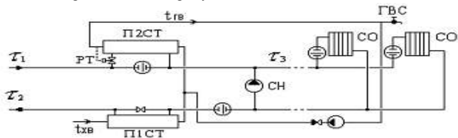
Рисунок 1.3.1 – Схема ЦТП
