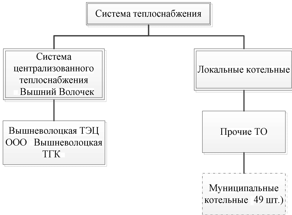
Рисунок 1.1.1 – Функциональная структура теплоснабжения на 01.01.2021 г.
